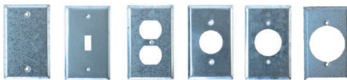
ปิดมิด (BLANK COVER) สวิทช์ (TOGGLE SWITCH) ปลั๊กคู่ (DUPLEX) ปลั๊กเล็ก (SINGLE RECEPTACLE) ปลั๊กกลาง (20A RECEPTACLE) ปลั๊กใหญ่ (POWER OUTLET)
